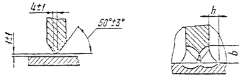
Чертеж 1, лист 2
