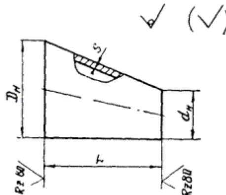
Переход эксцентрический
